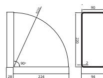
WYMIARY [MM]
