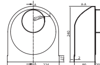
WYMIARY [MM]
