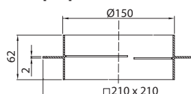
WYMIARY [MM]
