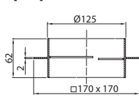
WYMIARY [MM]
