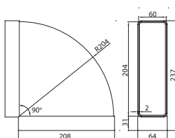
WYMIARY [MM]
