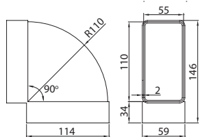
WYMIARY [MM]
