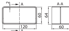
WYMIARY [MM]
