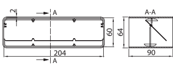
WYMIARY [MM]
