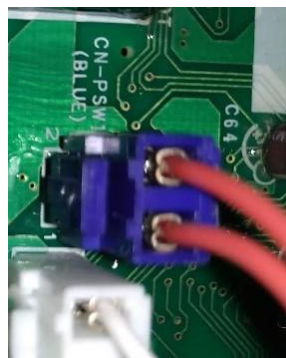
Złącze presostatu HP CN-PSW1
