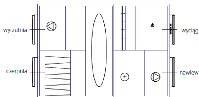
VUTR EH/WH EC Widok od strony serwisowej
