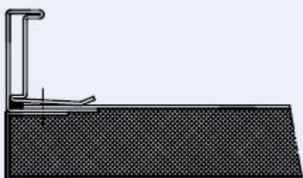
Izolacja dźwiękowa wewnętrzna wełną mineralną z powłoką niepylącą
