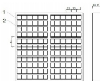
Rys. 2. Kratka prostokątna EI 120
